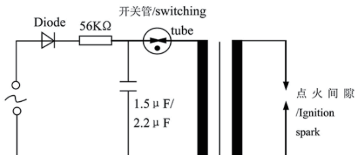
应用电路
